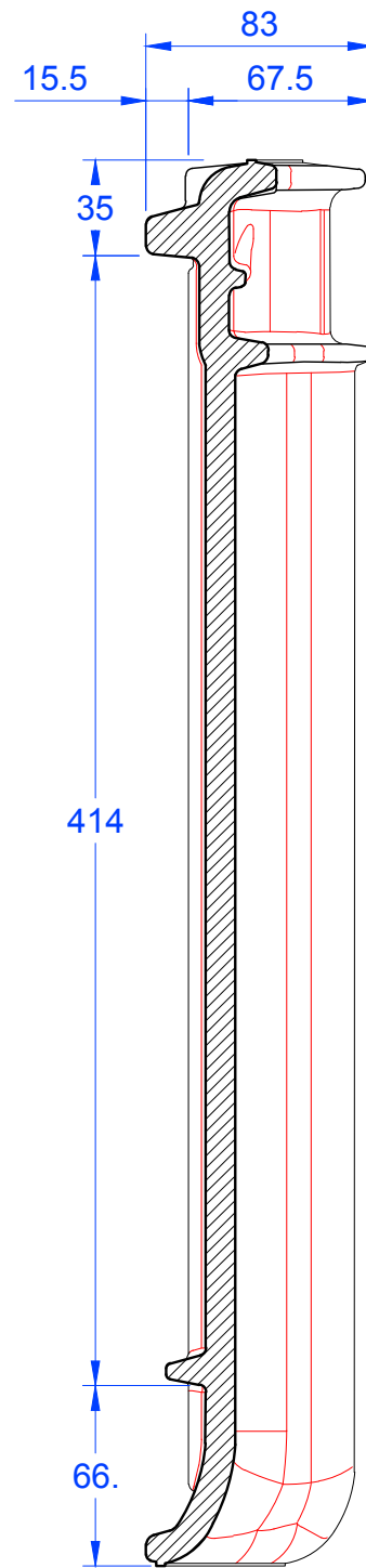
Schnitt B-B
