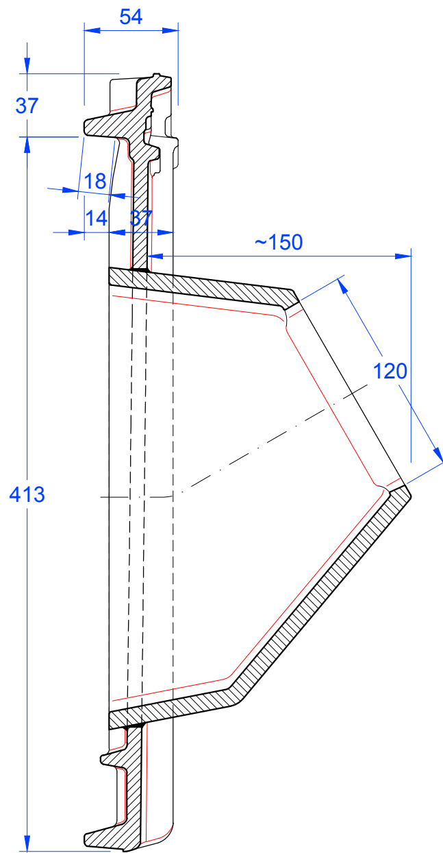
Schnitt B-B
