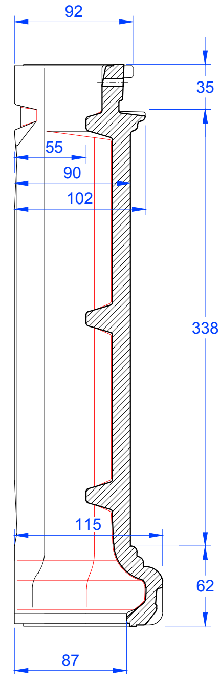
Schnitt A-A
