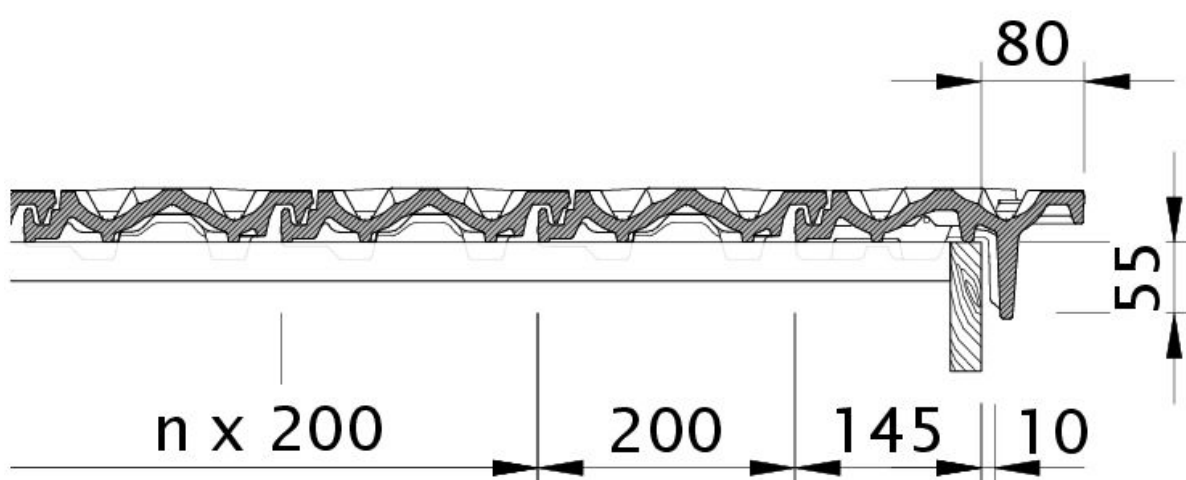
Tehnički crtež proizvoda RUSTICO OBL OBL
