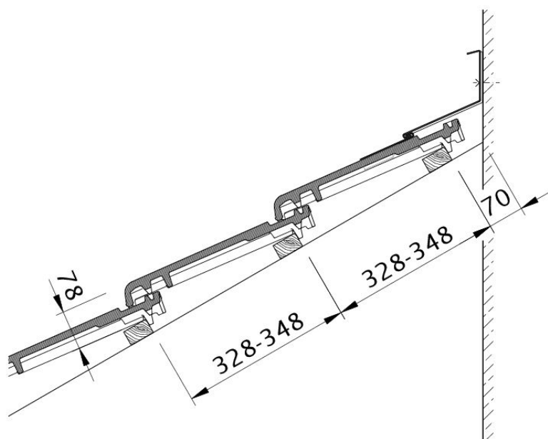
Tehnički crtež proizvoda RUSTICO WMF WMF
