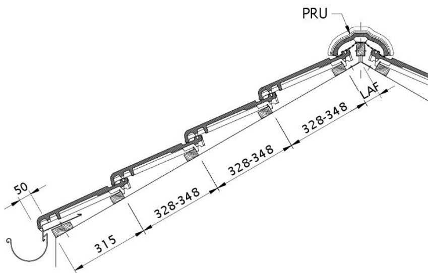
Tehnički crtež proizvoda RUSTICO DQF DQF
