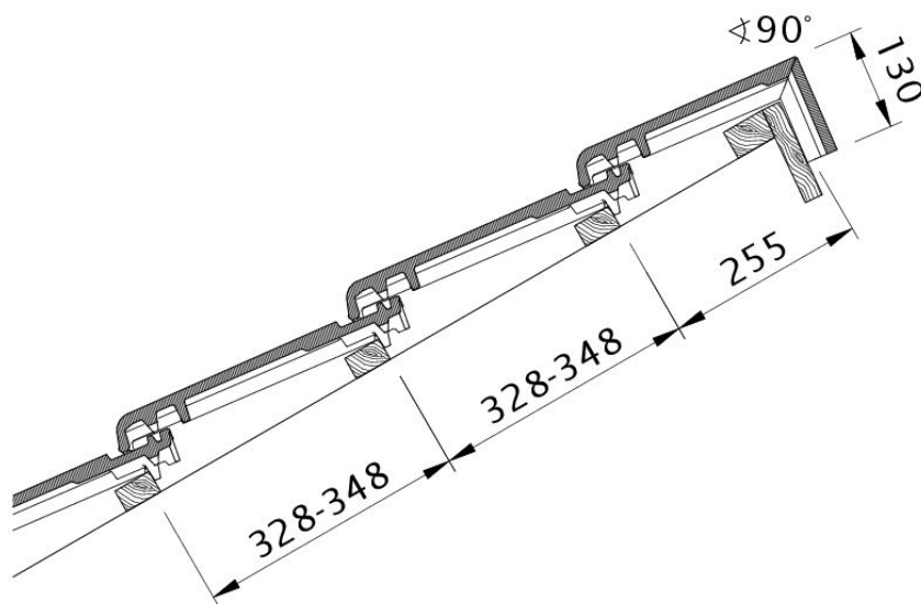
Tehnički crtež proizvoda RUSTICO PDA PDA
