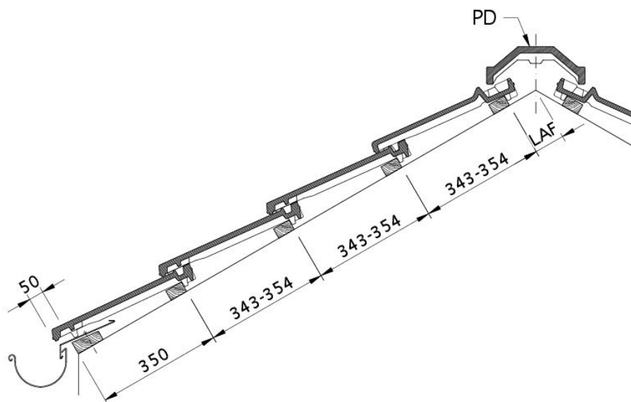
Tehnički crtež proizvoda DOMINO DQF DQF
